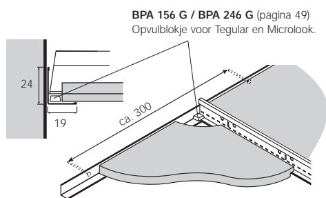
Standaard hoekafwerking met hoekprofiel BPT 1924 HD of BPT 1924 CA
