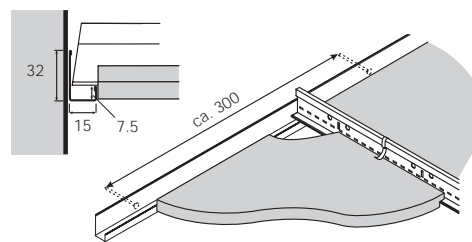
Afwerking met ongelijk U-profiel BPT 1575 HA
