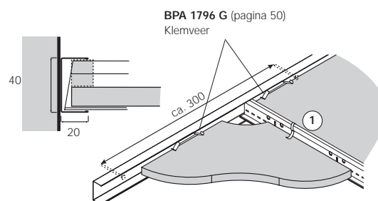
Afwerking met C-profiel BPT 2040 HA ① BPA 7890 G Universele klem
