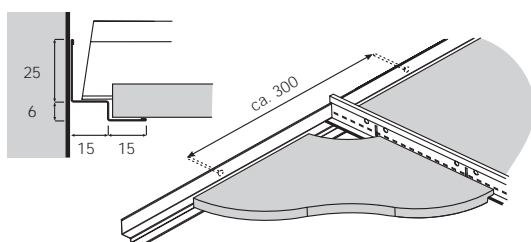
Afwerking met Schaduw hoekprofiel BPT 1506 H
