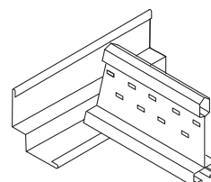
Profiel geknipt tot schaduwlijn BPT 1508 HB op hoeklijn
